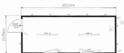
Prefabbricato modulare ad uso ufficio da 20' standard
